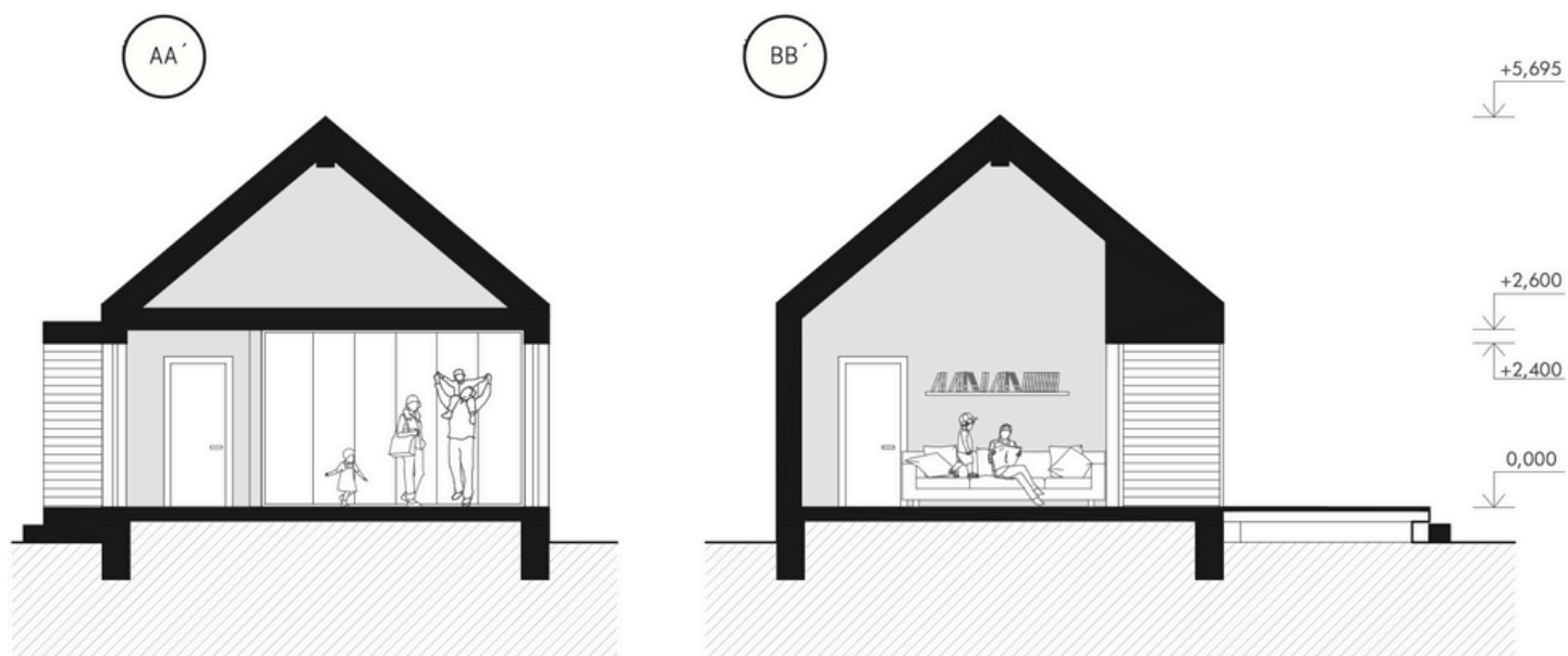
Řezy
